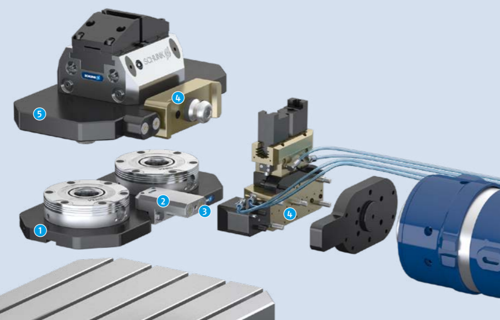
5 Automatisierte Werkstückbeladung.
